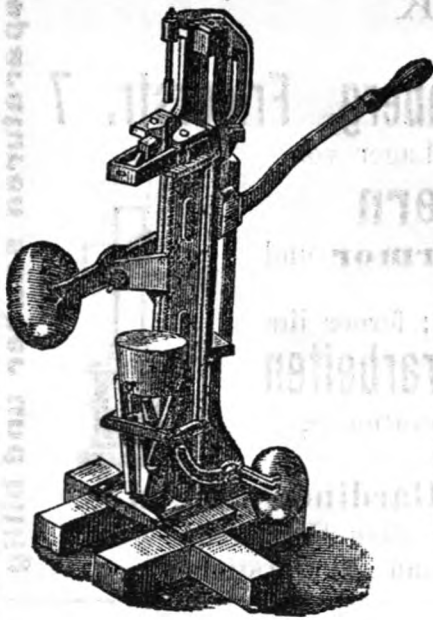
Verbesserte Flaschenkorbmachine.
