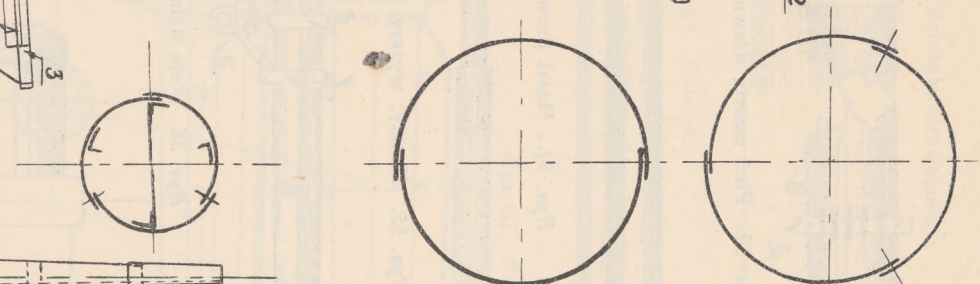
Rys.48. Poprzeczne przekroje żelaznych masztów i rei
