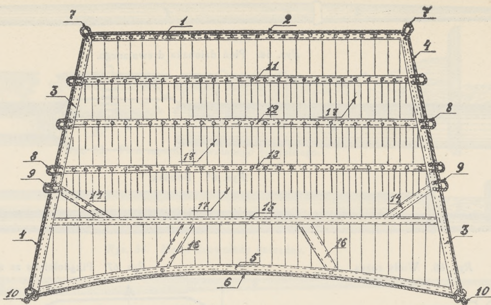
Rys. 71. Żagiel rejdowy.
