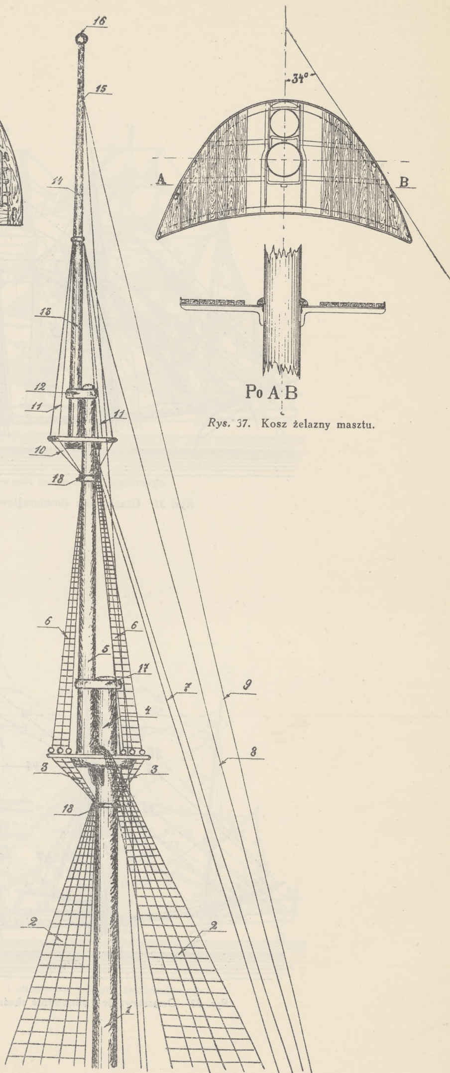
Rys. 33. Maszt dużego żaglowca.
