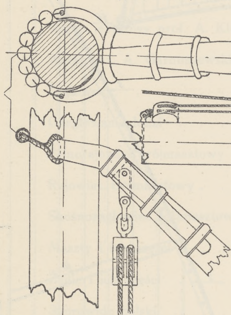
Rys. 66. Widły różca.
