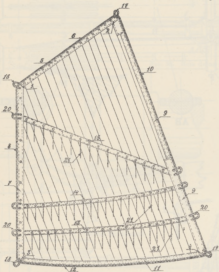
Rys. 72. Żagiel skośny
