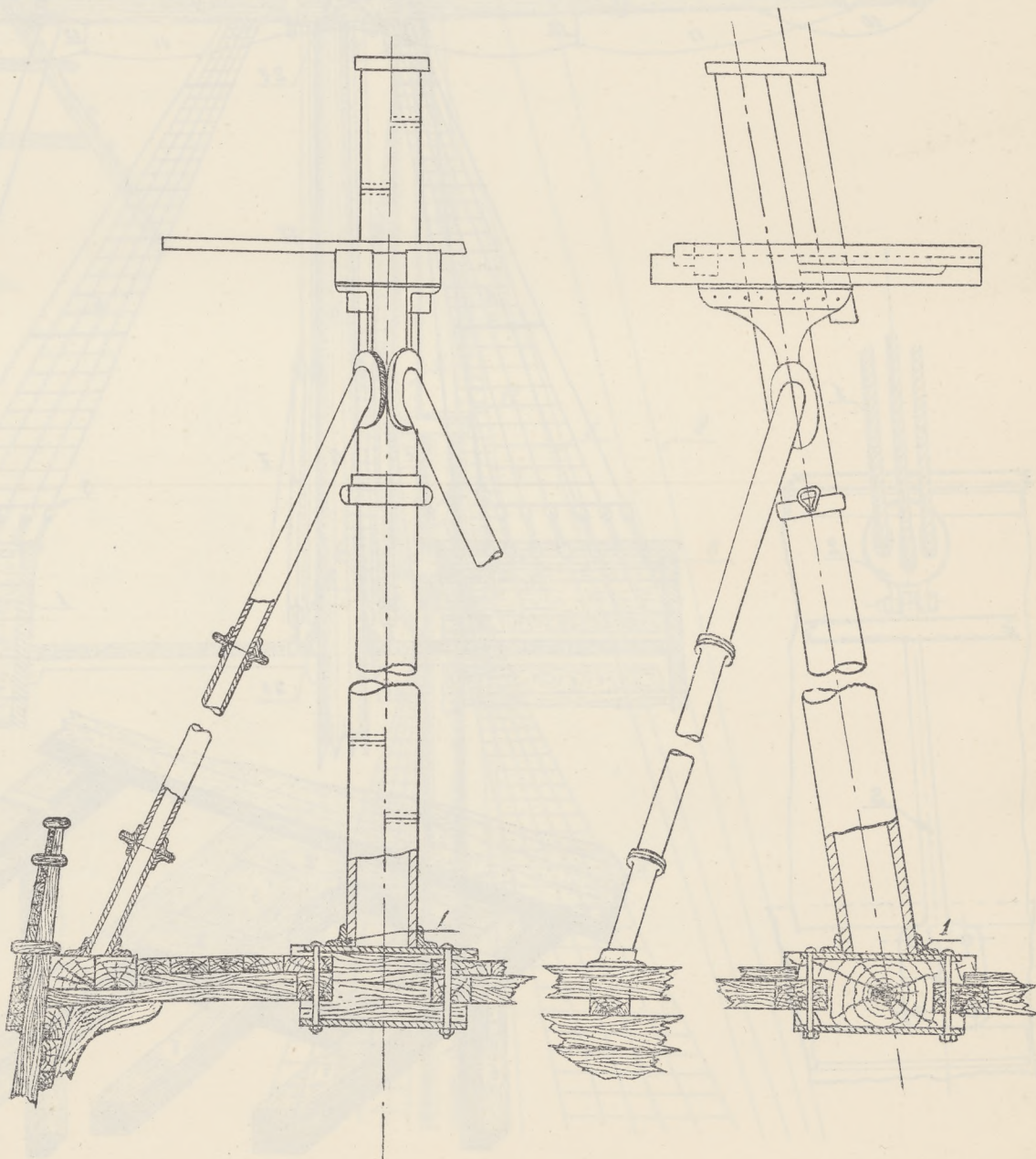
Rys. 44. Maszt trójnożny.
