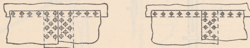
Rys.51. Złącza blach rei żelaznej (stalowej)
