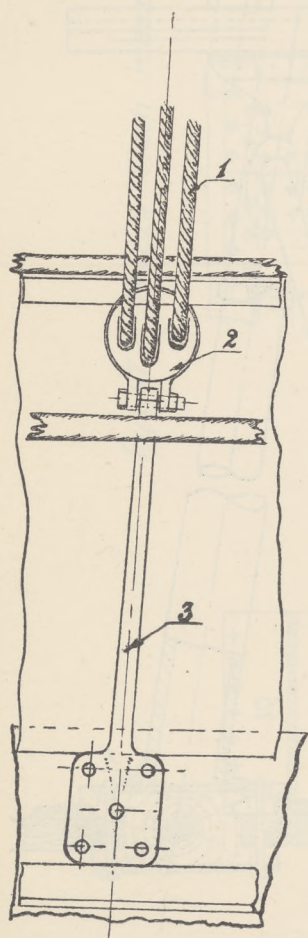
Rys. 41. Podwiesz burtowa i nawlek ściągu.
