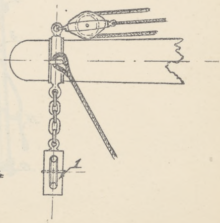
Rys. 70. Pik żórawia przymasztowego.
