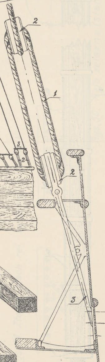
Rys. 40. Ściągacz wieży masztu i podwiesz burtowa.
