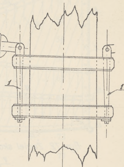
Rys. 68. Pięta i sworzeń żórawia przymasztowego lub dolniaka.
