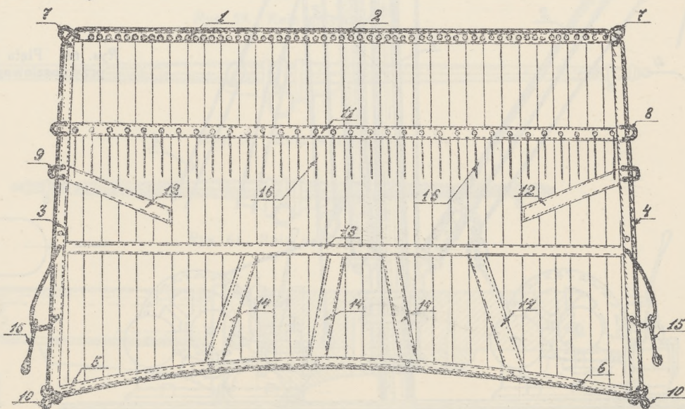
Rys. 74. Żagiel rejdowy dolny.
