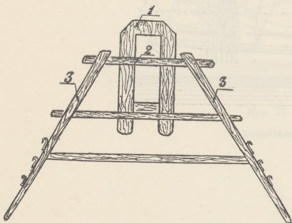
Rys. 35. Siodło masztu.
