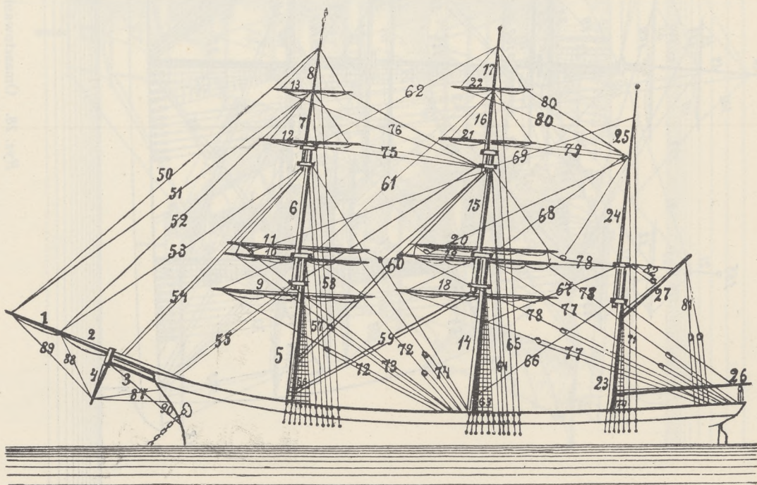
Rys. 30. Omasztowanie i olinowanie rejewca trójmasztowego.
