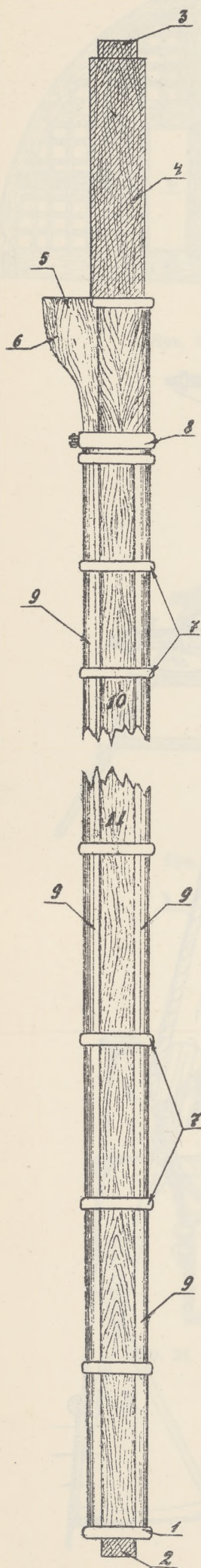
Rys. 42. Pień masztu drewnianego złożonego.
