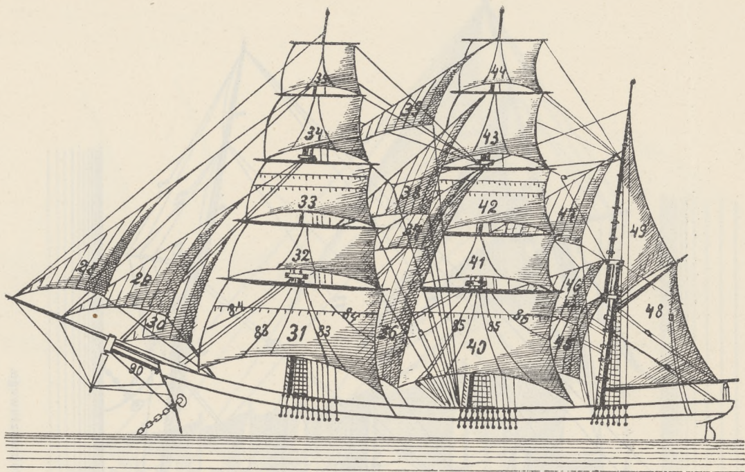
Rys. 29. Ożaglowanie rejewca trójmasztowego.
