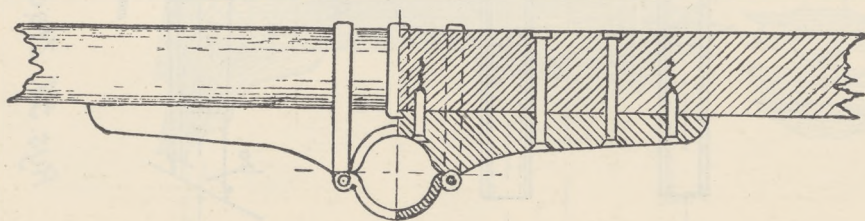
Rys. 62. Wieżba rej górnych.
