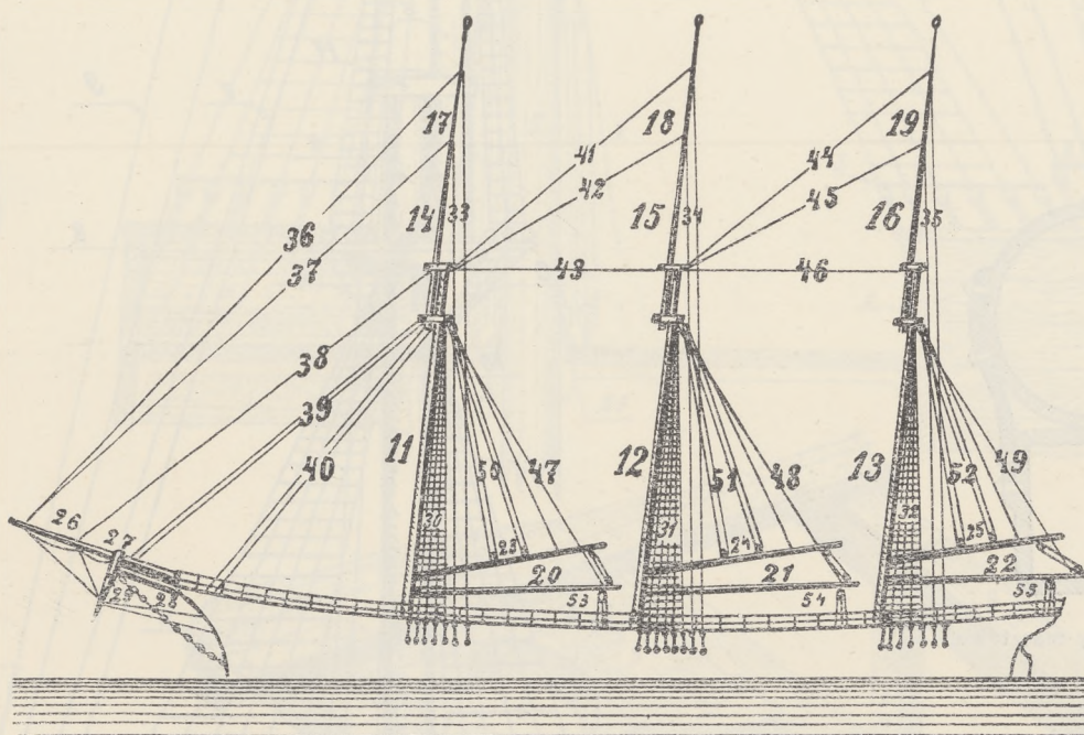
Rys. 32. Omasztowanie i olinowanie skośnożaglowca trójmasztowego.
