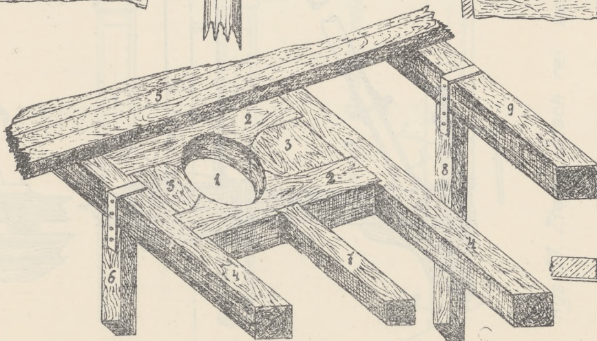
Rys. 39. Więzba masztu.
