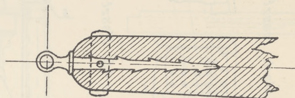
Rys. 58. Wieżba dolniaka.
