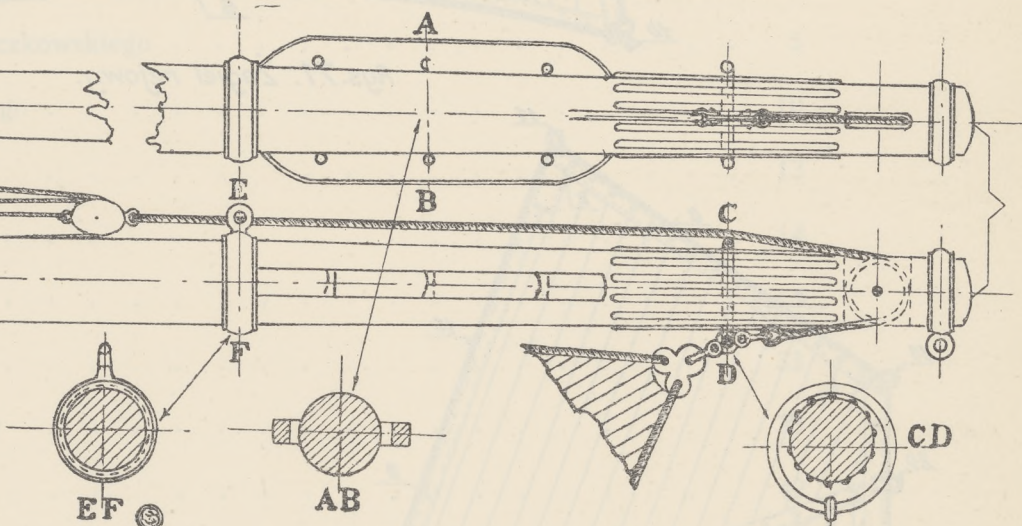
Rys. 67. Pik dolniaka ze skrótnicą.
