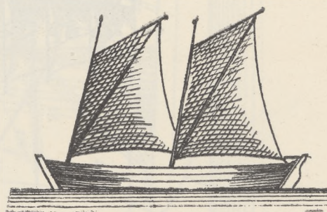
Rys. 26. Ożaglowanie prętowe.
