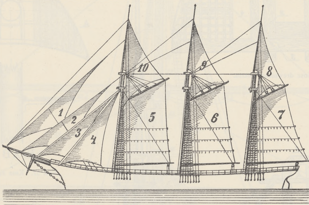
Rys. 31. Ożaglowanie skośnożaglowca trójmasztowego.
