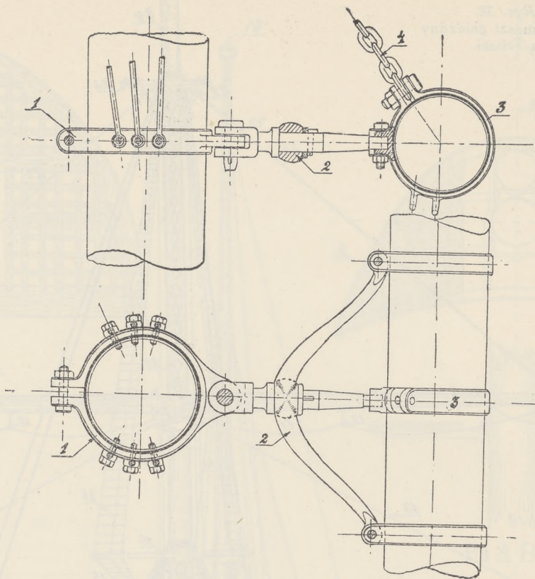
Rys. 43. Pierścień i więzba rejowa.
