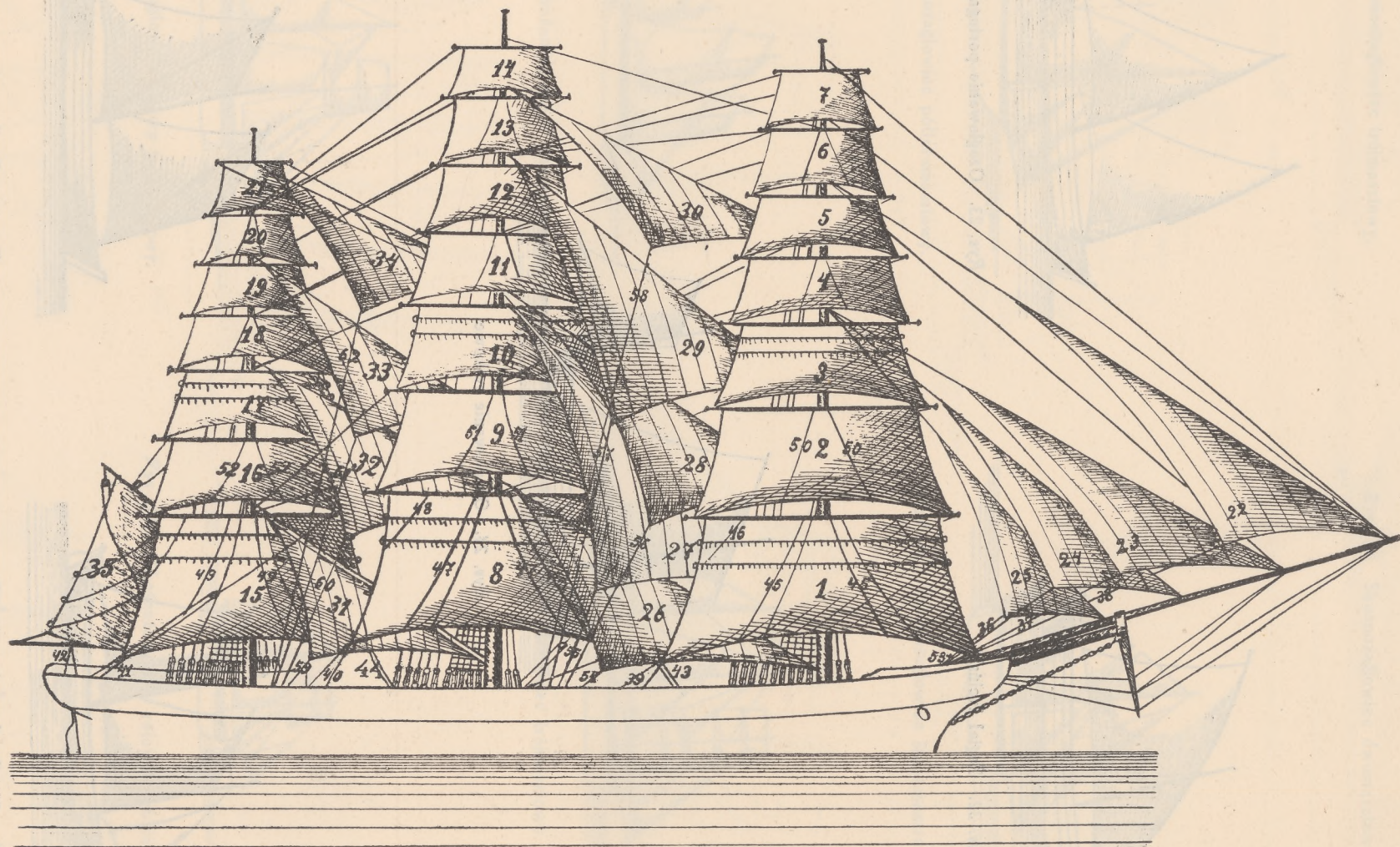
Rys. 27. Ożaglowanie pełnorejowca trójmasztowego.
