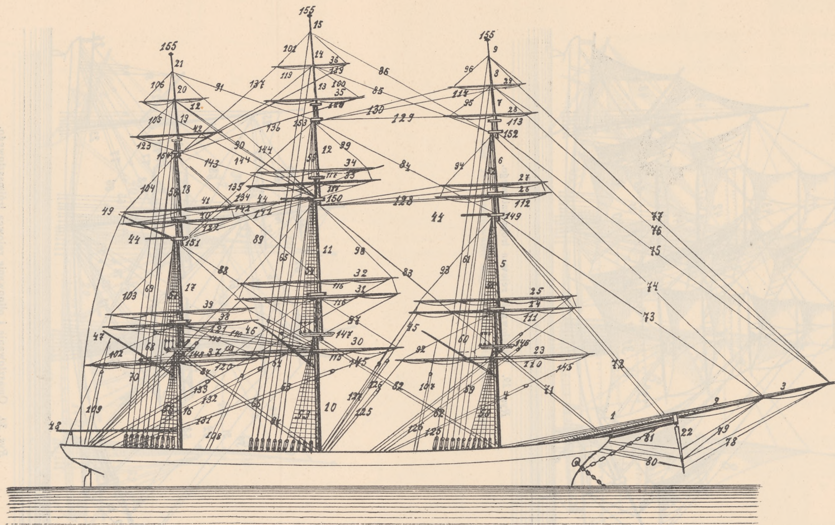
Rys. 28. Omasztowanie i olinowanie pełnorejowca trójmasztowego.
