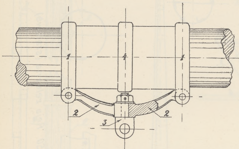
Rys. 57. Wieżba rej dolnych.
