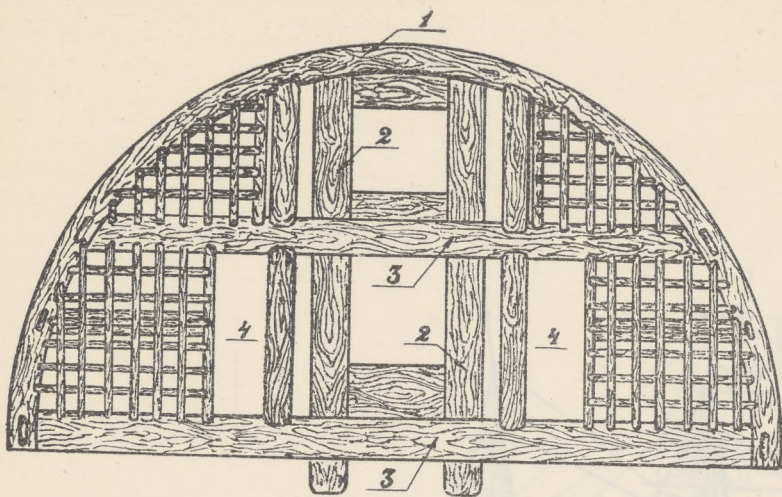
Rys. 34. Kosz drewniany masztu.
