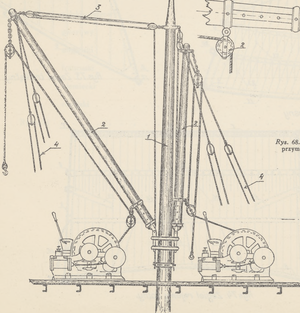
Rys. 69. Żórawie przymasztowe.
