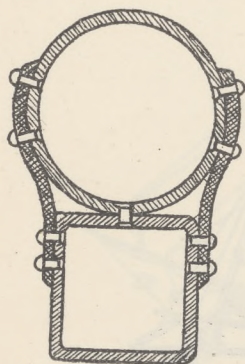
Rys. 36. Dyby masztowe.
