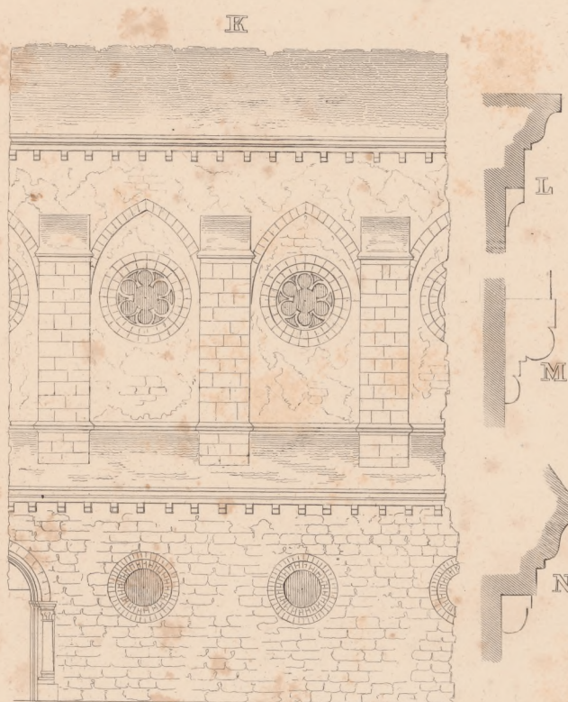
Ansicht von e bis f.
