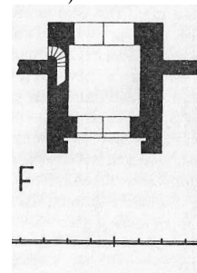
Plan bramy ze schodami w Nowej Marchii – 8 F
